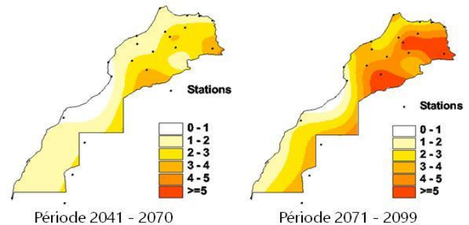
Projections climatiques des températures comparées à celles de la période 1961-1990
