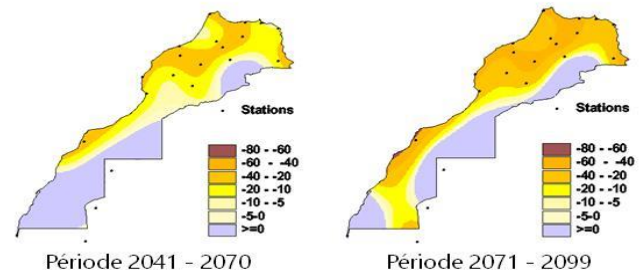
Projections climatiques des précipitations comparées à celles de la période 1961-1990
