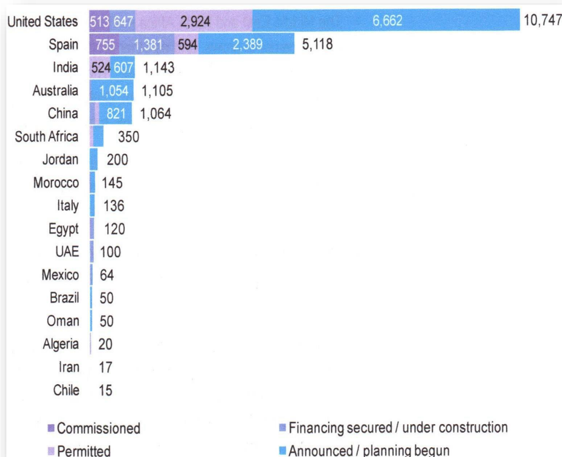
Graphique n°7 : Projets CSP dans les pays leaders à fin T2 2011 (en MW)
