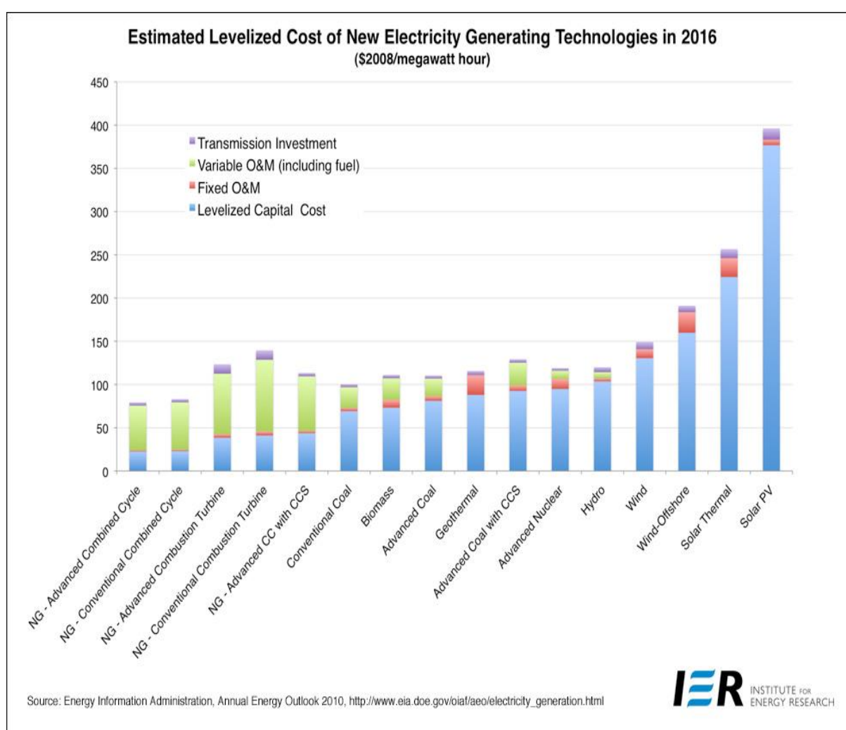
Graphique n°6 : Coûts des nouvelles technologies de génération de l'électricité
